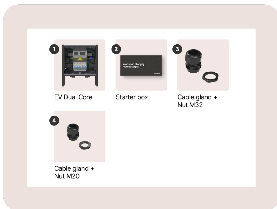
Afbeelding 1: inhoud van de doos met de kernassemblage voor een socketmodel
