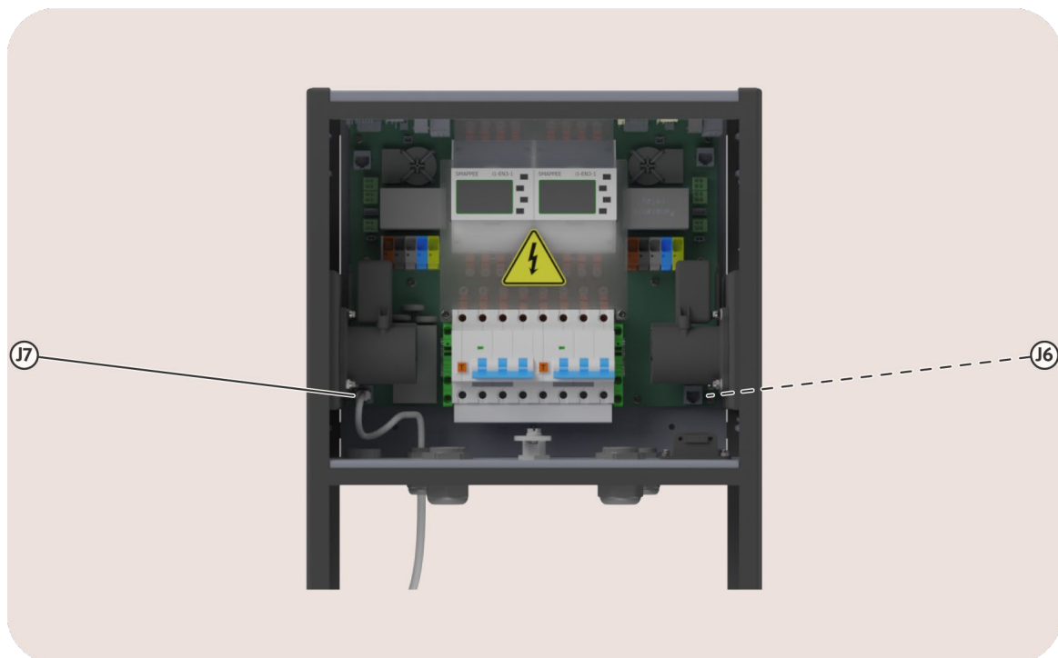
Afbeelding 36: poort J7 voor internetinvoer en poort J6 voor optionele serieschakeling
