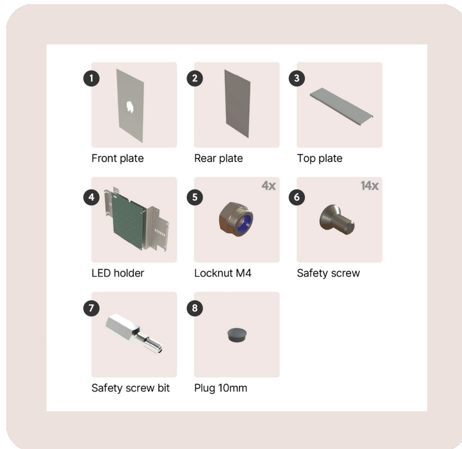
Afbeelding 4: inhoud van de doos met de platen
